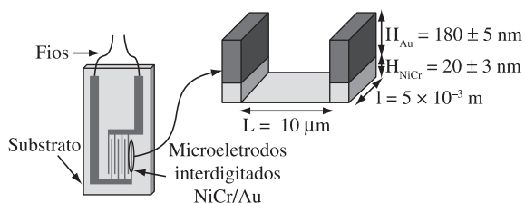
Figura 1. Representação esquemática da estrutura dos microeletrodos interdigitados utilizados para as caracterizações elétricas dos filmes. H_{Au} e H_{NiCr} são, respectivamente, as espessuras das camadas de NiCr e de Au, enquanto L e l a distância média e o comprimento dos eletrodos.
