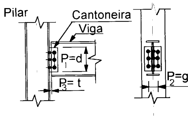
(a) ligação com cantoneiras duplas de alma (Tipo DA).
