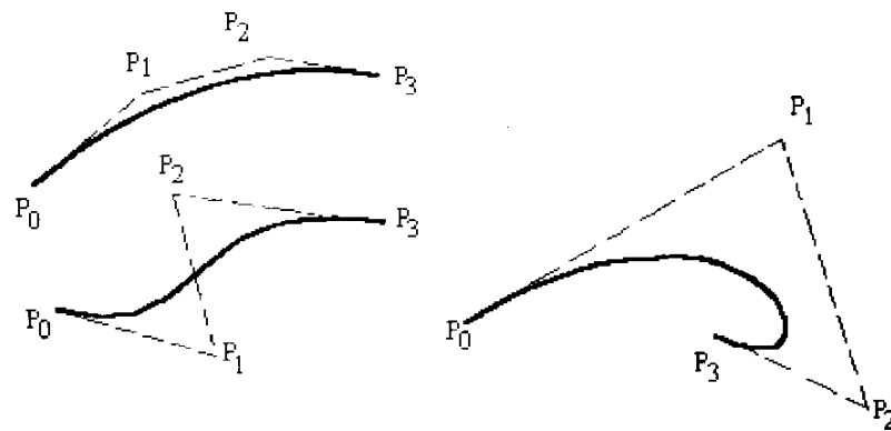
Figura II.4 - Curvas de Bézier P_0 \dots P_3 ; são os pontos que formam o polígono de controle.
