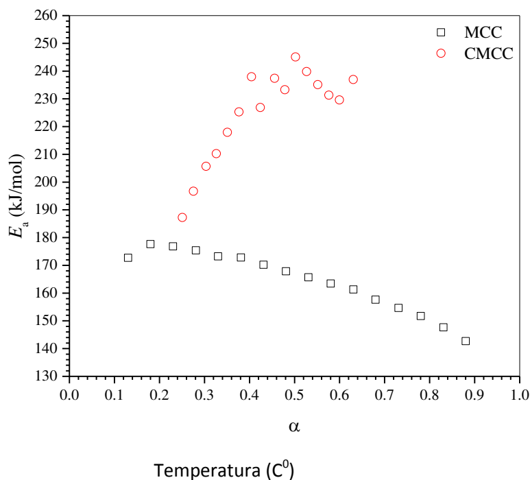
Figura 7. Gráfico da energia de ativação de Arrhenius para a decomposição térmica da celulose MCC e para a celulose modificada com ácido de Meldrum MCCM
