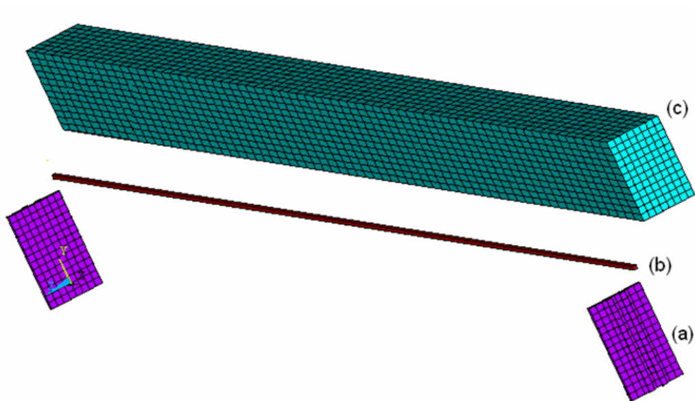
(a) chapa de topo, (b) tirante de aço e (c) viga de madeira.
