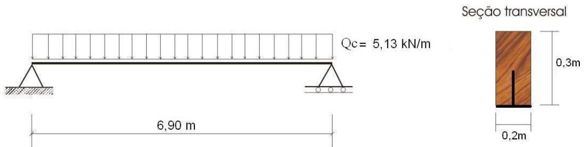
Figura 6. 5 – Modelo da viga mista, perfil T de aço e madeira com o carregamento aplicado
