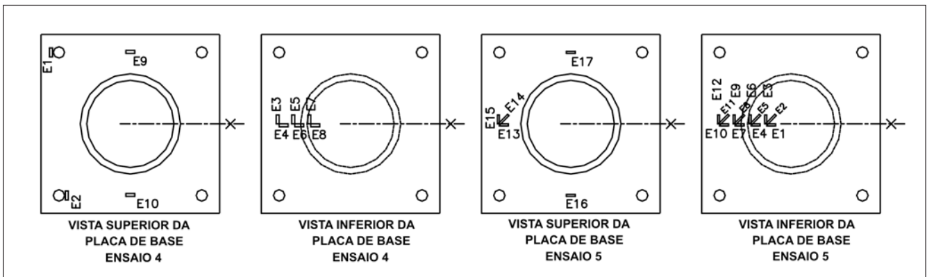
Figura 3 - Esquema de instrumentação com extensometria - Ensaios 4 e 5.
