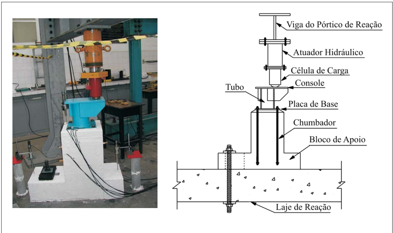
Figura 1 - Esquema geral de montagem dos ensaios.
