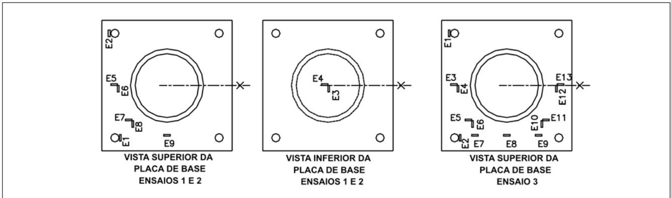
Figura 2 - Esquema de instrumentação com extensometria - Ensaios 1, 2 e 3.
