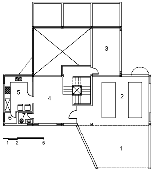
Figura 4.4 - Projeto arquitetônico: planta do terceiro e quarto pavimento FONTE: Arquivo escritório de arquitetura
