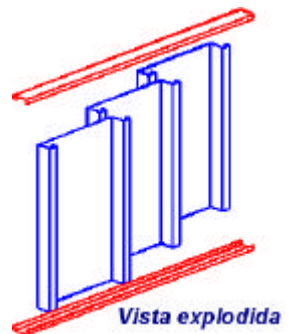
Figura 3.11 - Formação do painel – FONTE: Disponível em: http://www.metalica.com.br/pg_dinamica/bin/pg_dinamica.php?id_pag=564 Acesso em jan. 2004.
