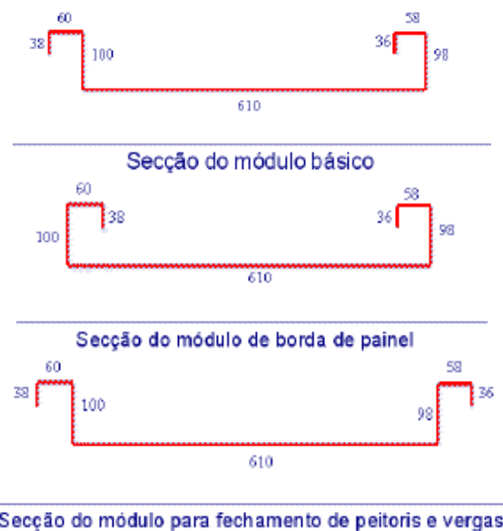
Figura 3.9 - Seções típicas dos módulos – FONTE: Disponível em < http://www.metallica.com.br/pg_dinamica/bin/pg_dinamica.php?id_pag=564 > Acesso em jan. 2004.
