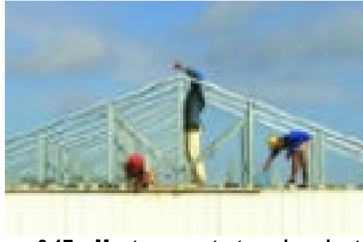
Figura 3.17 – Montagem estrutura da cobertura. FONTE: Disponível em: < http://www.casafortemedabil.com.br > Acesso em jan. 2004.
