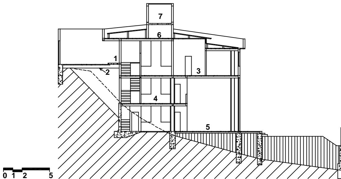
Legenda: (1) N+0,10 – Garagem/Hall, (2) N-0,50 - Jardim, (3) N-1,16 - Suítes, (4) N-4,40 - Escritório, (5) N-7,64 - Convívio, (6) N+2,96 - Boiler, (7) N+4,66 – Cx D'Água
