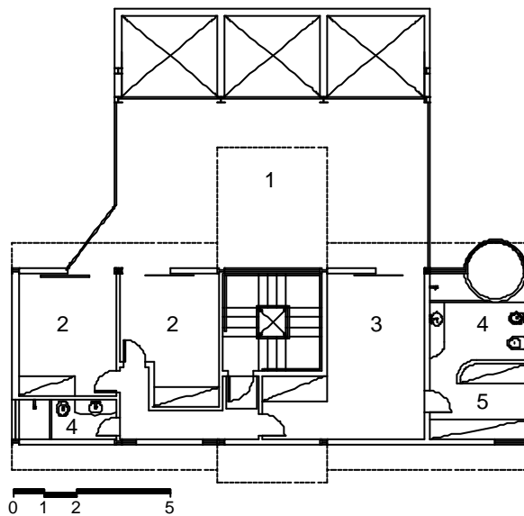
Figura 4.5 – Projeto arquitetônico: planta do quinto pavimento FONTE: Arquivo escritório de arquitetura
