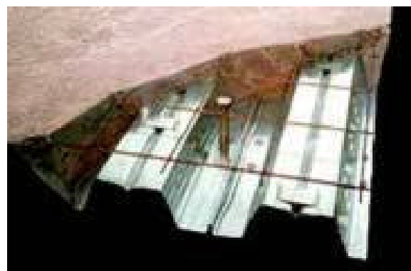
Figura 3.31 – Detalhe composição de laje steel deck - FONTE: Disponível em: < http://www.metlica.com.br/pg_dinamica/bin/pg_dinamica.php?id_pag=538 > Acesso em jun. 2005.
