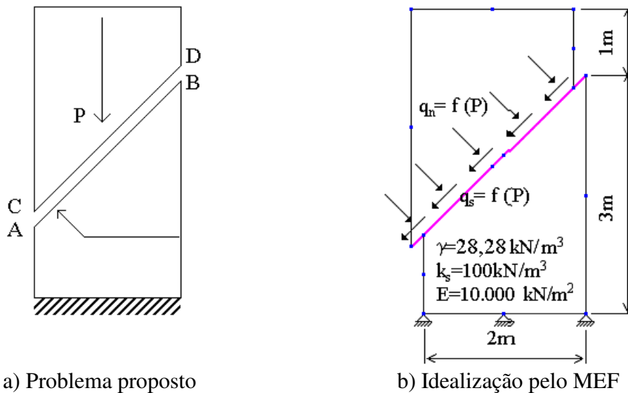
Figura 4.9 – Bloco deslizando sobre outro bloco com interface inclinada.
