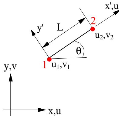
Figura 3.2 – Elemento de Barra B2.
